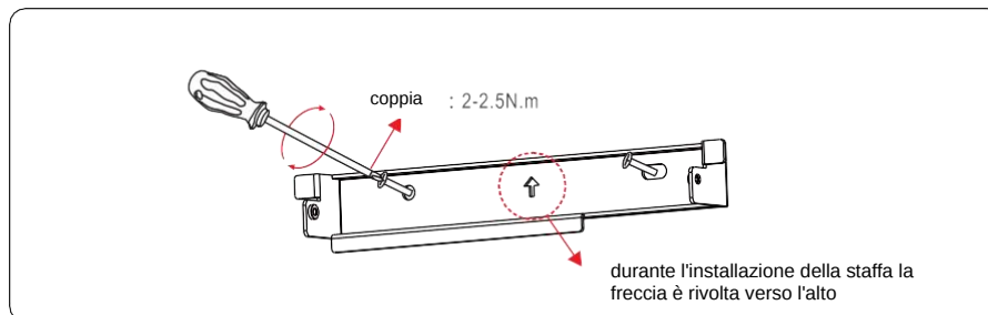
Figure 4.13 installazione del pannello posteriore
