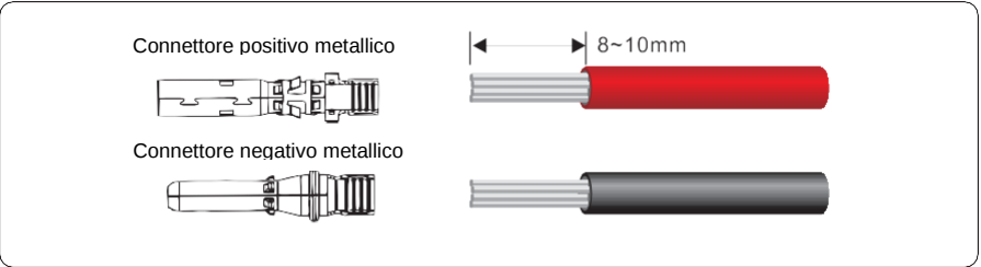
Figure 5.10 Rimozione dello strato isolante dal cavo DC (unit: mm)
