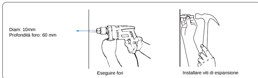
Figure 4.12 Perforare i fori e installare l'espansione (unit: mm)
