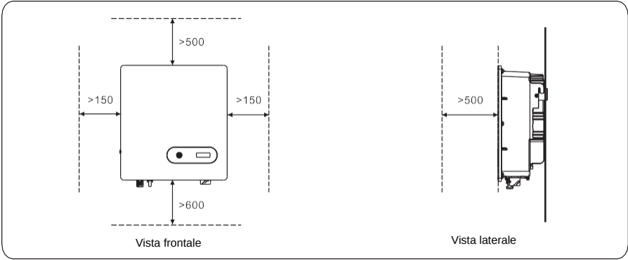
Figure 4.4 requisiti spazio installazione (unit: mm)
