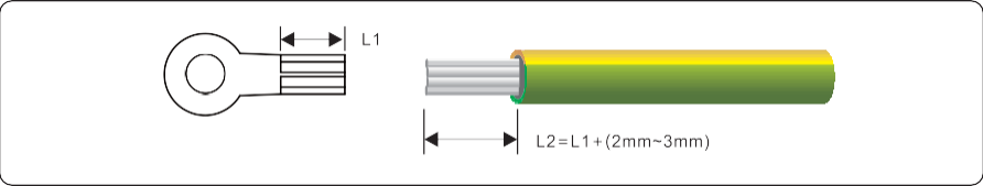
Figure 5.1 Lunghezza esposta (unit: mm)
