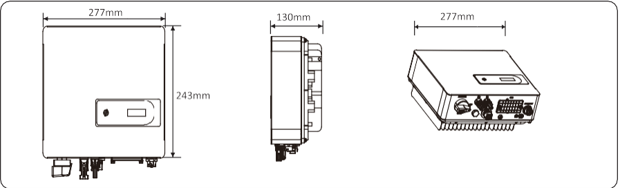
Figure2.3 1.5K-3.6K Inverter fotovoltaico con ingresso singolo MPPT (unit: mm)
