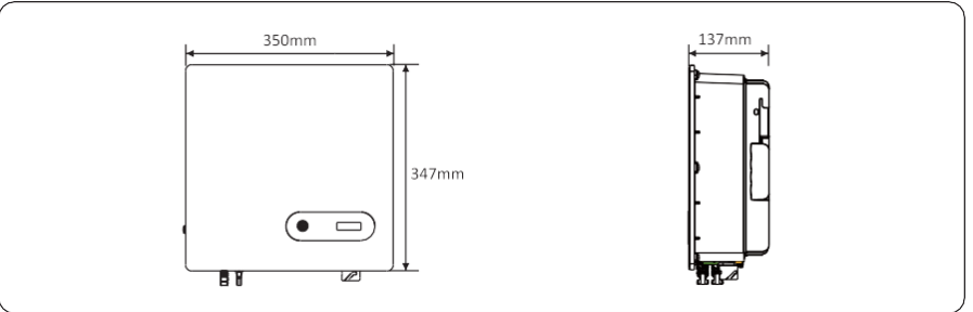
Figure2.4 4K-6K Inverter fotovoltaico con doppio ingresso MPPT (unit: mm)
