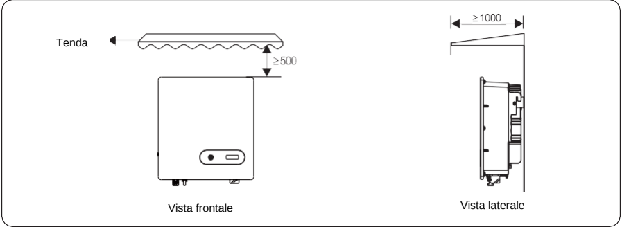
Figure 4.3 Ambiente di installazione con tenda (unit: mm)
