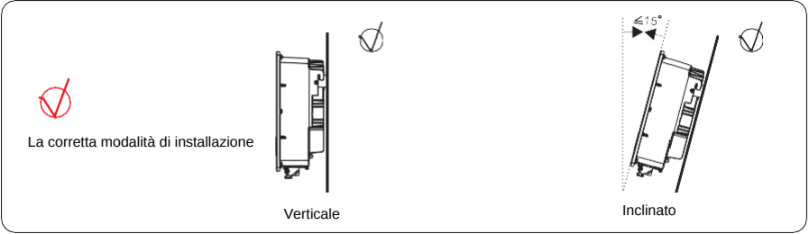
Figura 4.8 Corretta modalità di installazione
