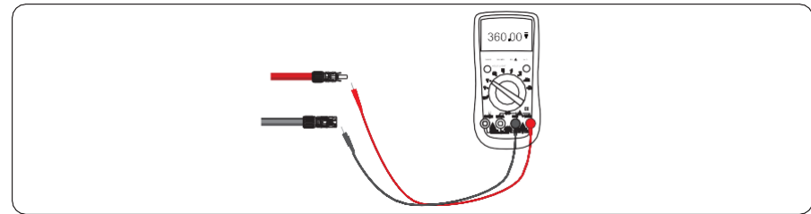
Figure 5.14 Controllo della tensione di ogni Stringa
