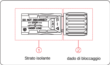
Figure 5.9 Composizione connettori negativi
