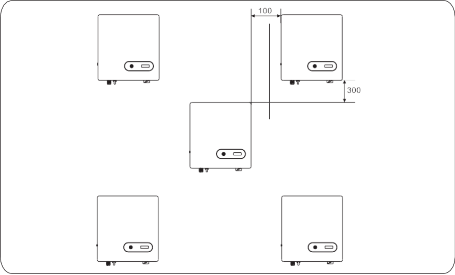
Figure 4.6 Installazione modalità triangolo (unit: mm)
