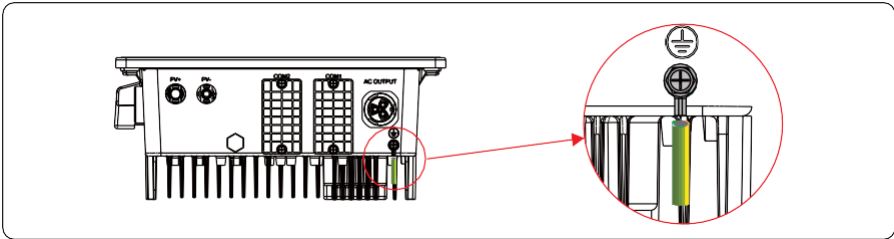
Figure 5.4 Fissare il cavo PGND
