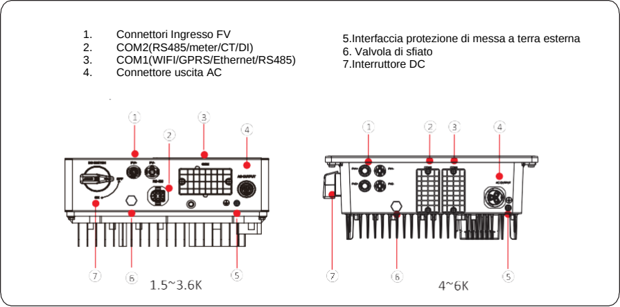
Figure 2.6 La vista posteriore di questa serie di inverter
