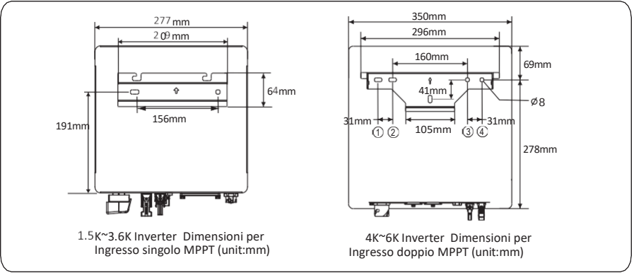
Figure 4.10 Determinare le posizioni per praticare i fori (unit: mm)
