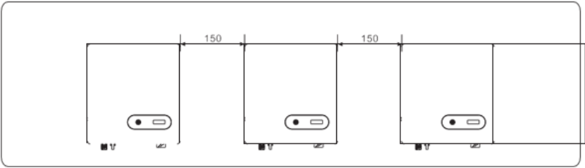
Figure 4.5 Installazione lungo la stessa linea (unit: mm)
