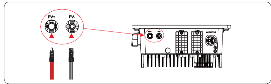
Figure 5.15 Collegamento all'inverter
