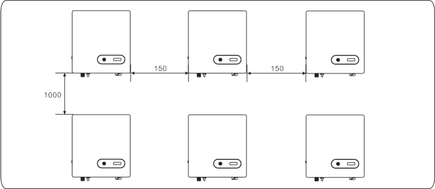
Figure 4.7 Installazione modalità impilata (unit: mm)
