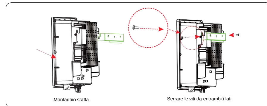
Figure 4.14 Fissaggio dell'inverter
