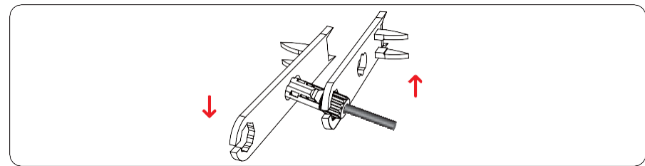
Figure 5.13 Serraggio Connettori
