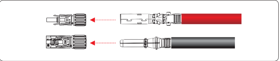
Figure 5.12 Collegamento di connettori positivi e negativi
